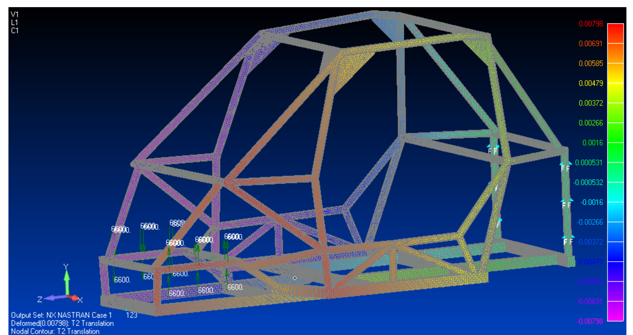
Figura 5: Análise MEF.
